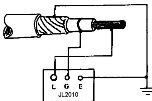
屏蔽电缆绝缘测试接线图
